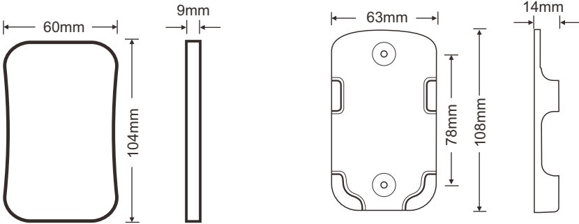
遥 控 器
