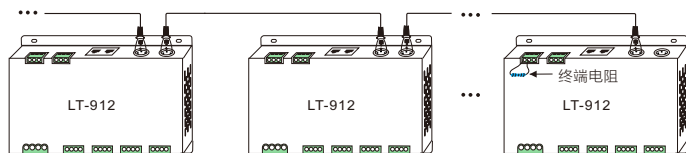
3针XLR并联连接
