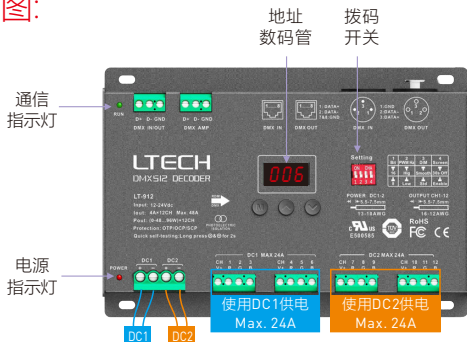
拨码开关
