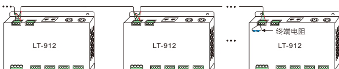
绿色端子并联连接
