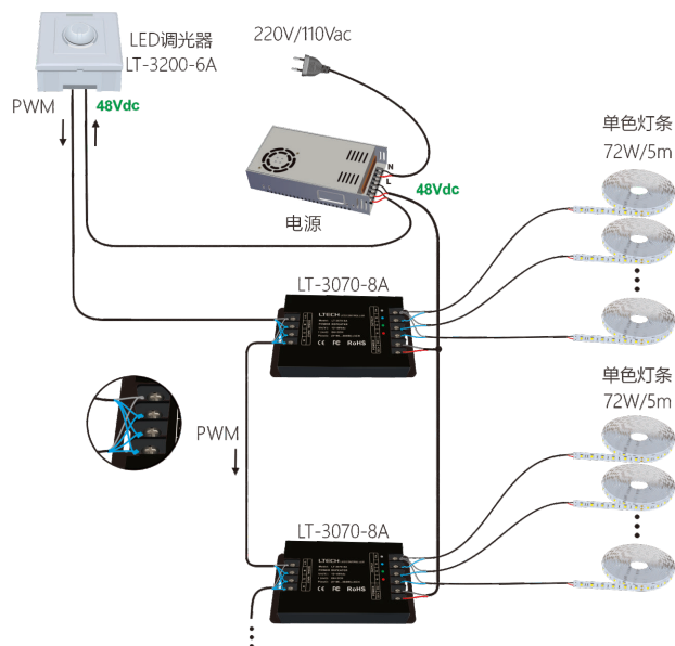
3. 下图为LED调光器连接恒压功率扩展器示意图
