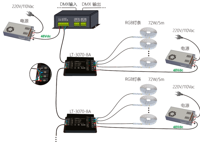
3. 下图为LED调光器连接恒压功率扩展器示意图
