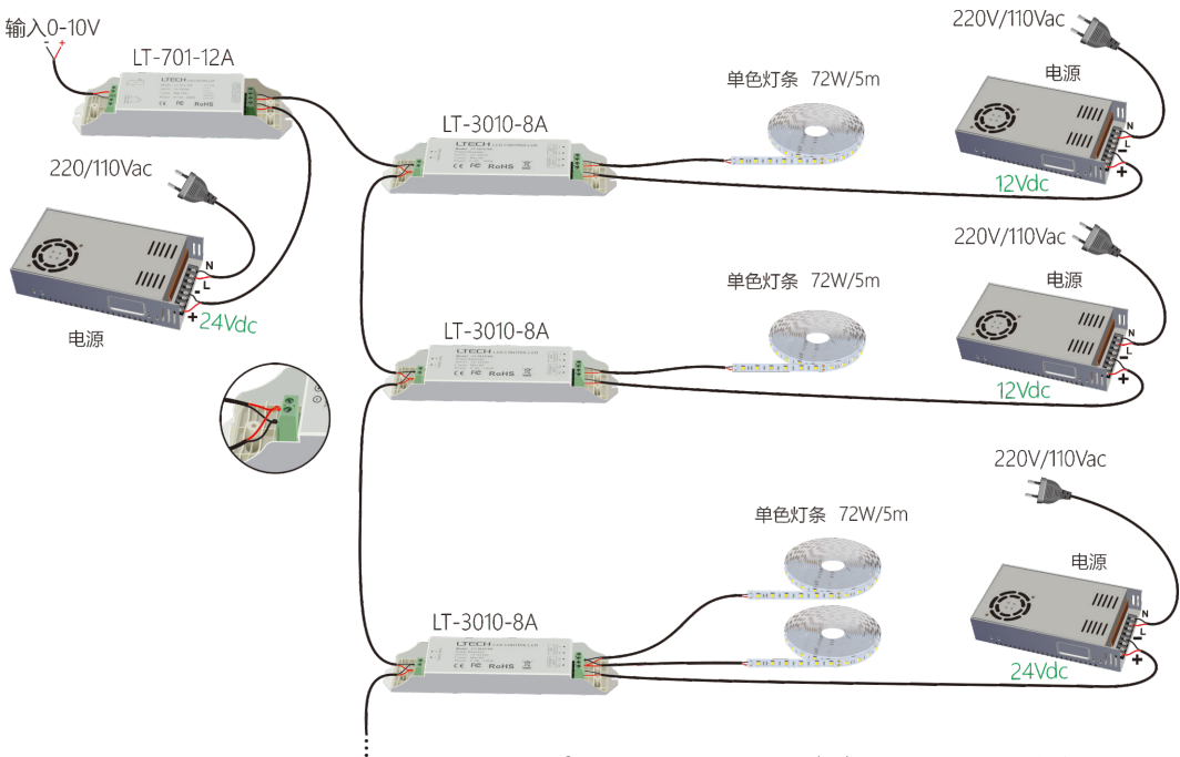
与LED调光驱动器连接
