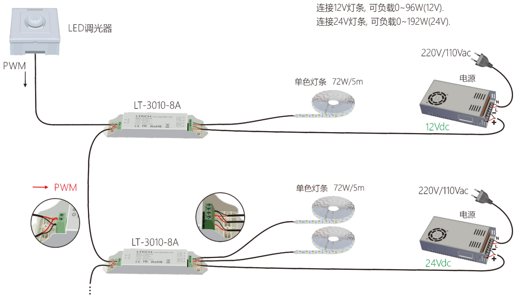
与LED调光驱动器连接
