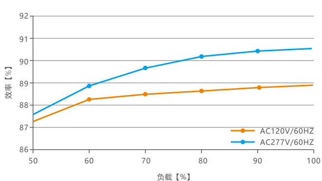
效率与负载关系图
