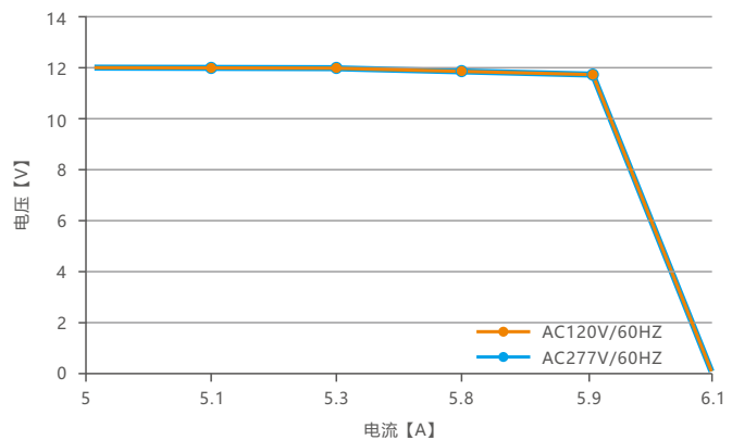
过载曲线
