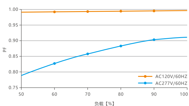
功率因数特征图
