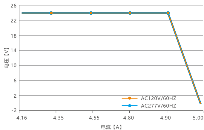
过载曲线
