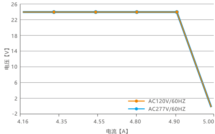
过载曲线
