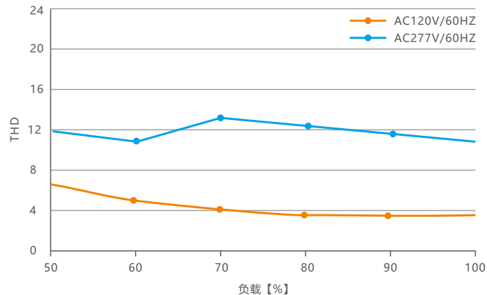
THD与负载关系图
