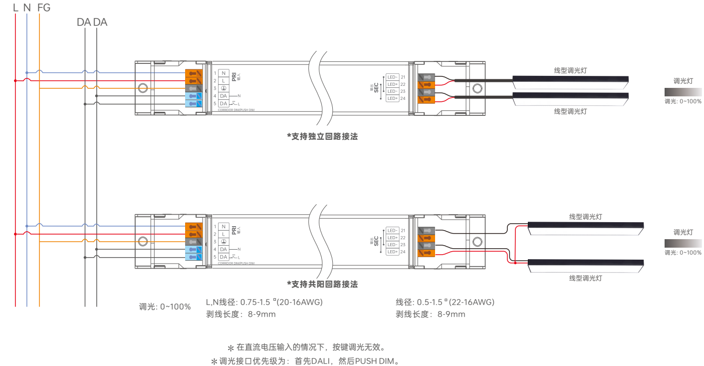
接线图
